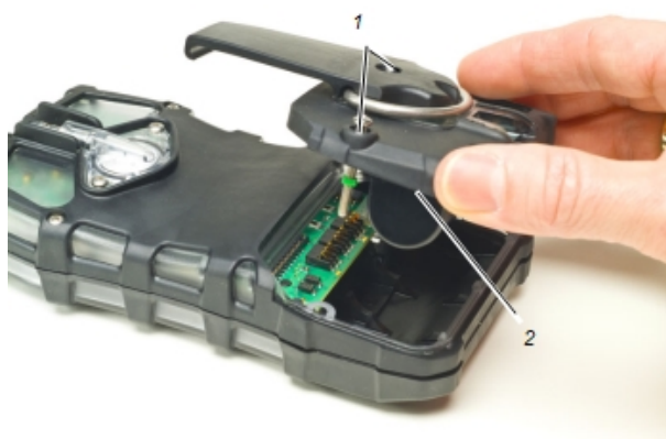
Figura 13 Substituição da bateria
